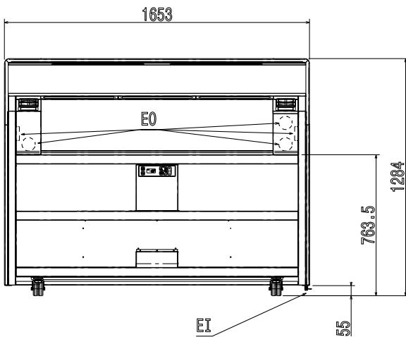
Oldalnézet
